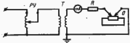
РУ —регулирующее устройство; T —трансформатор; R —сопротивление 0,5 МОм; B —образец из карбо- лита с нанесенной пленкой испытуемой эмали.
